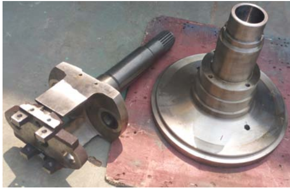
Shaft of horizontal ring die pellet mill
